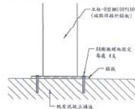
H型鋼立柱施作斷面示意圖 S=NTS
