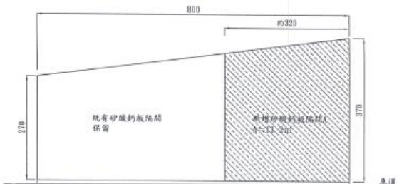
b-b 斷面示意圖 S=1:60
