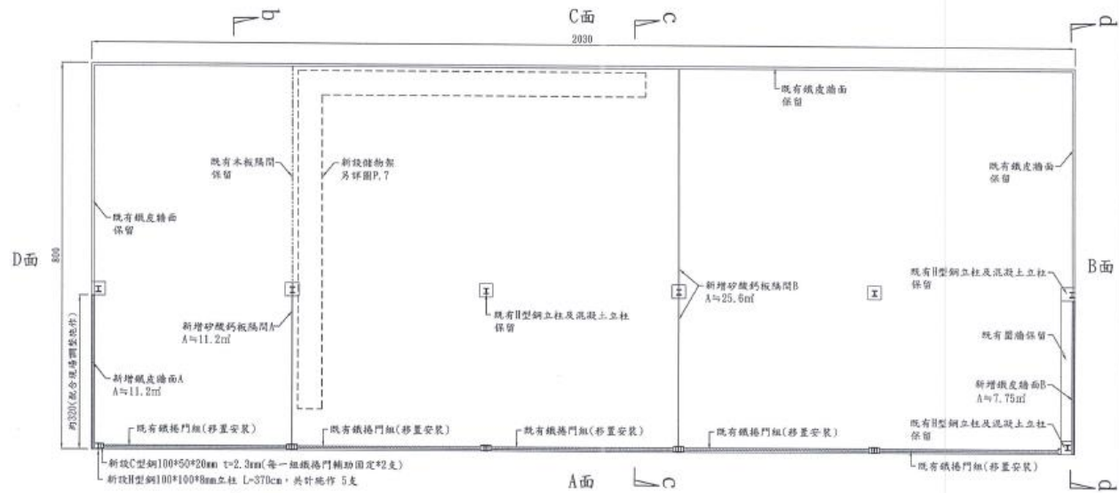
清潔隊儲藏室配置平面示意圖 S=1:60
