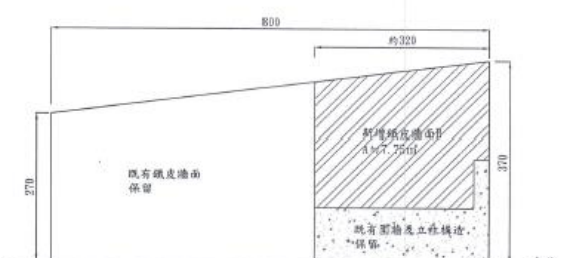
d-d 斷面示意圖 S=1:60
