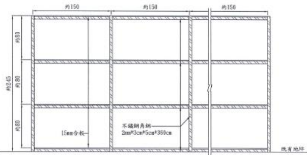
新設儲物架立面示意圖 S=1:30
