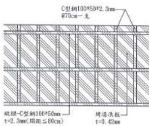
新增鐵皮牆面施作斷面示意圖 S=NTS
