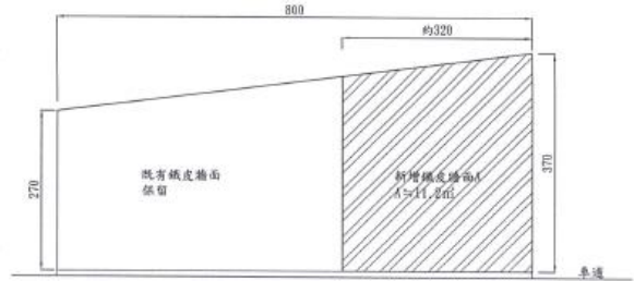
清潔隊儲藏室配置D面立面示意圖 S=1:60
