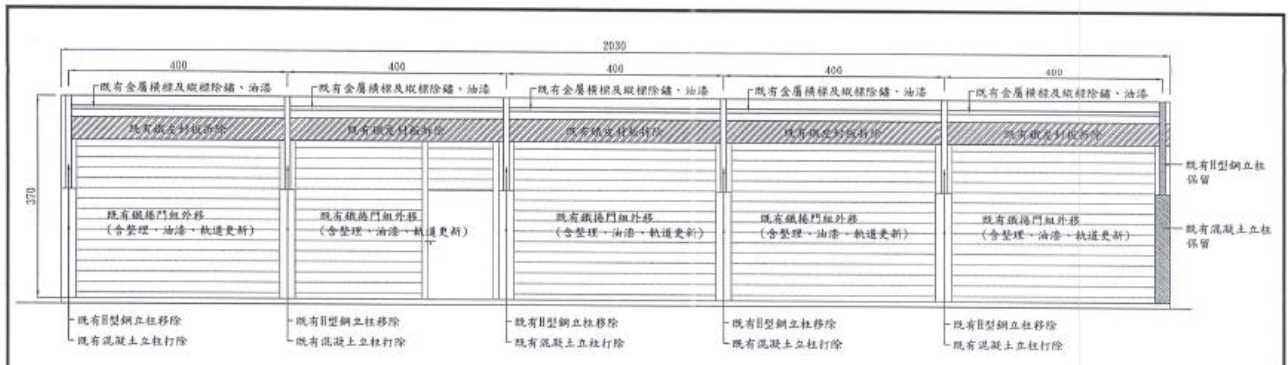
清潔隊儲藏室A面現況立面示意圖 S=1:60
