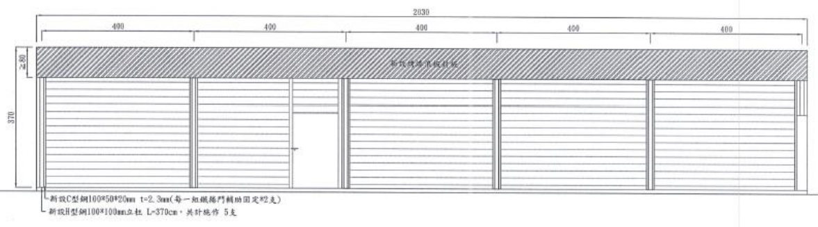
清潔隊儲藏室A面配置立面示意圖 S=1:60
